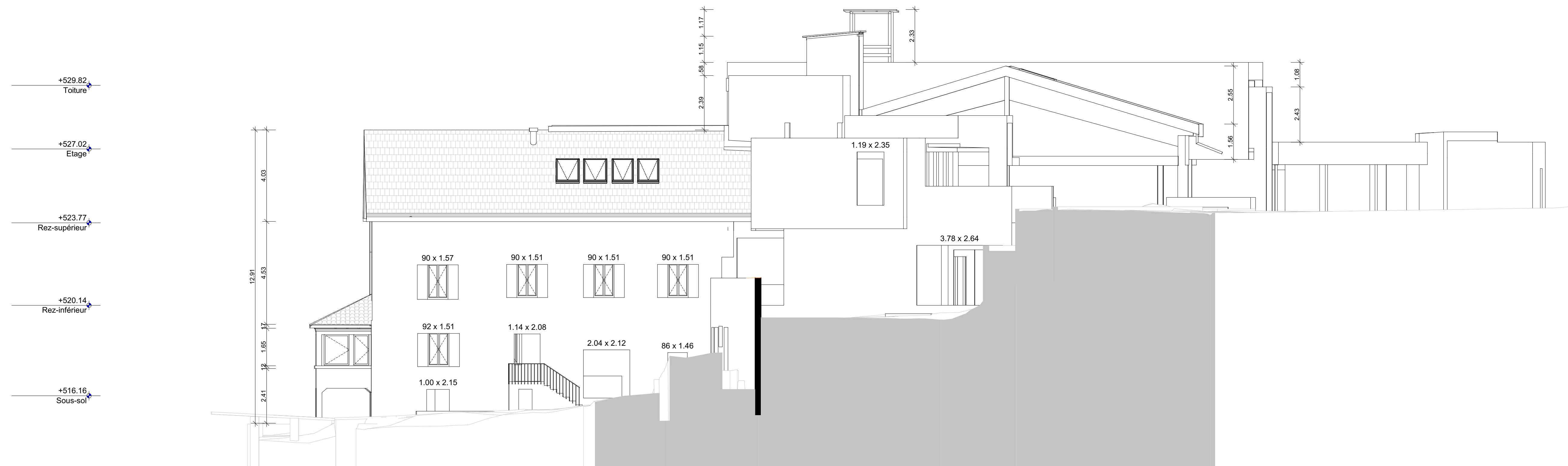
FAÇADE OUEST 1/100
