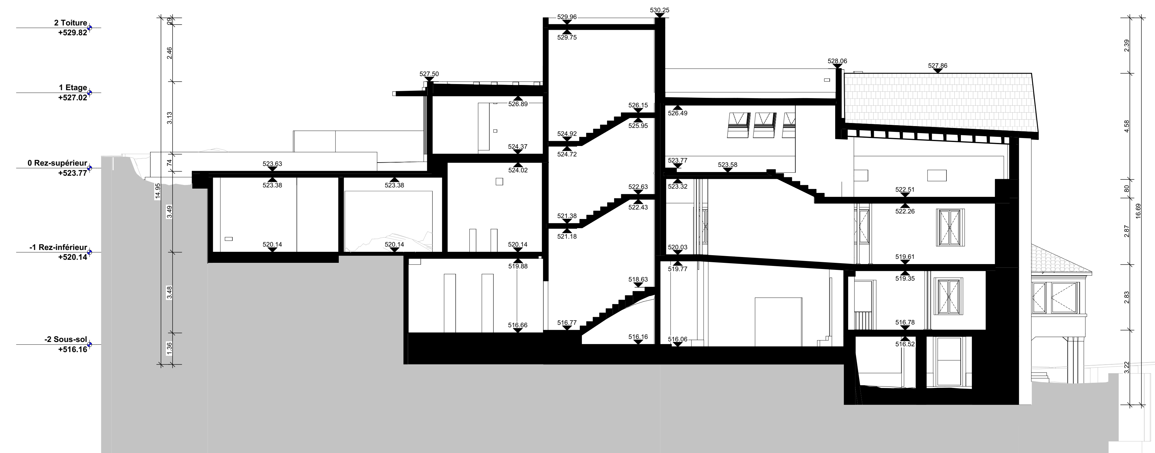
COUPE B-B 1/100
